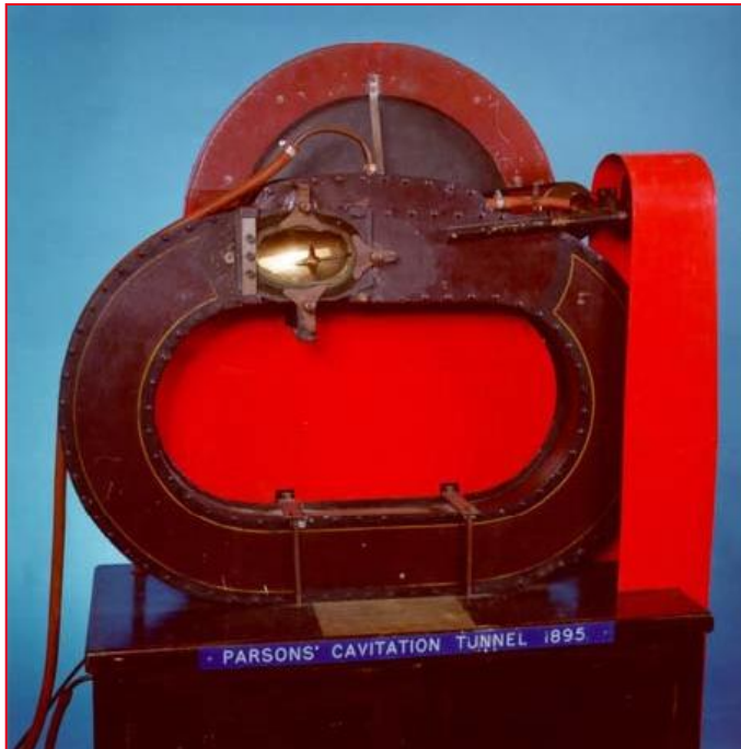
Erster Kavitationskanal gebaut von Sir Charles Parsons (1895)
